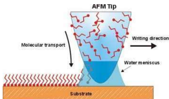
Figure 3: Principe de fonctionnement du DPN
