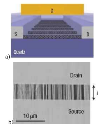
Figure 18: a) Représentation schématique d'un transistor à base de nanotubes alignés (S source, D drain, G grille). b) Image du dispositif au microscope électronique à balayage (L représente la longueur du canal).
