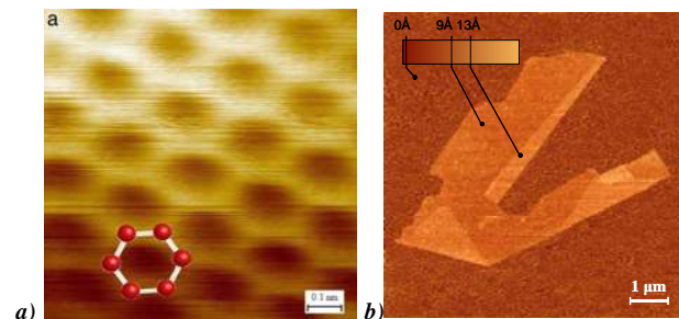
Figure 12: a) Observation au microscope à effet tunnel (STM) d'une monocouche de graphène l b) Feuille de graphène visualisée au microscope à force atomique, la zone pliée possède une hauteur de 4 Å soit celle d'une monocouche de graphène.
