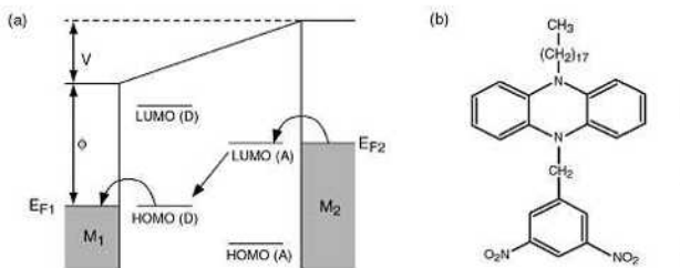
Figure 9: Redresseur de courant moléculaire formé par l'association d'un motif donneur d'électrons (D) et d'un motif accepteur d'électrons (A), séparés par un motif isolant ( \sigma ). Gauche : Diagramme énergétique du composant. Sous une faible tension appliquée dans le sens passant, le niveau de Fermi de la cathode ( EF_2 ) monte et celui de l'anode ( EF_1 ) descend légèrement. Les électrons peuvent circuler entre la cathode et la LUMO de l'accepteur, puis entre l'HOMO du donneur et l'anode.
